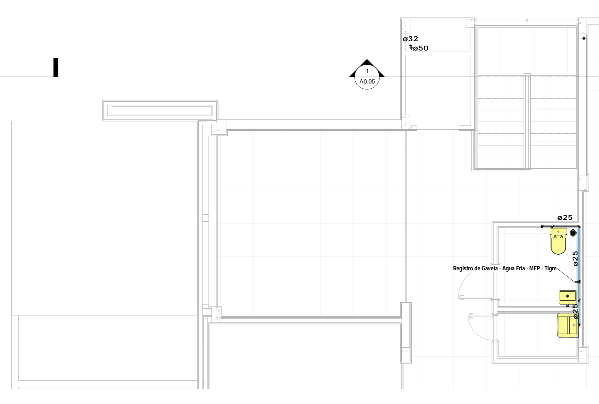
2 01.AF.PAVIMENTO SUPERIOR 1:50
