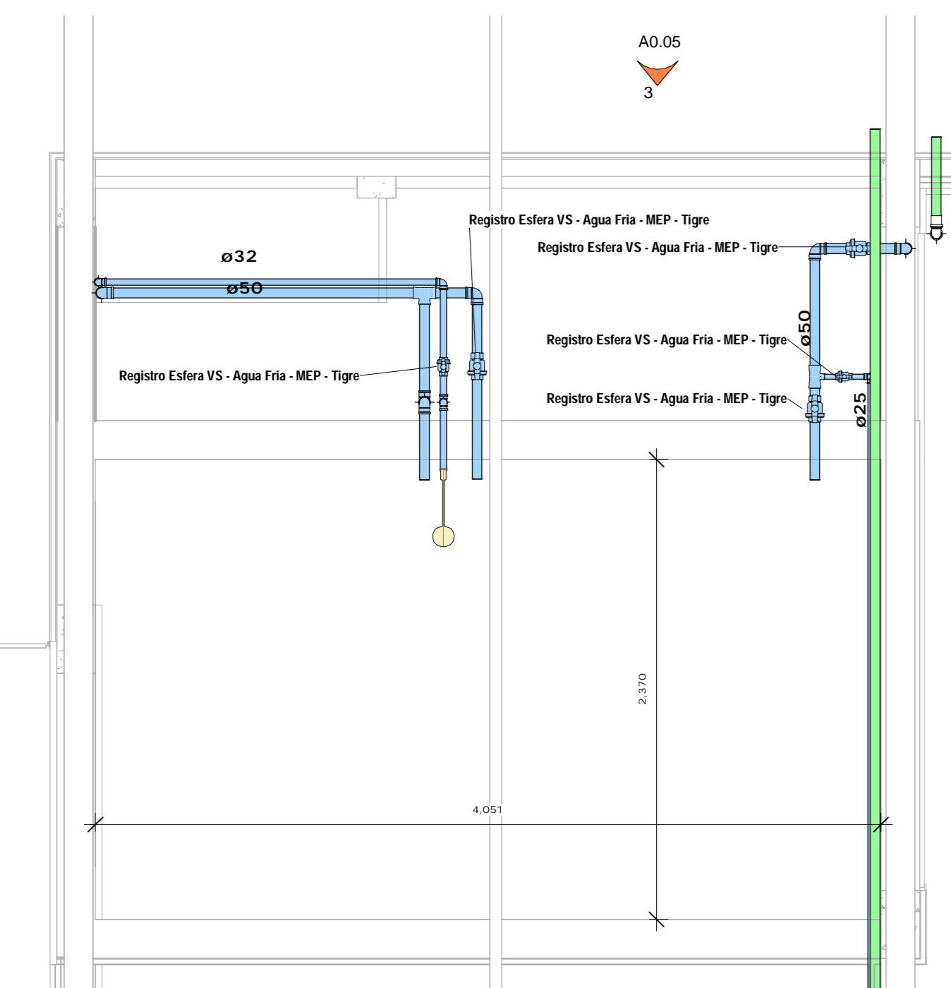
3 02.AF.CAIXA D'AGUA 1:25
