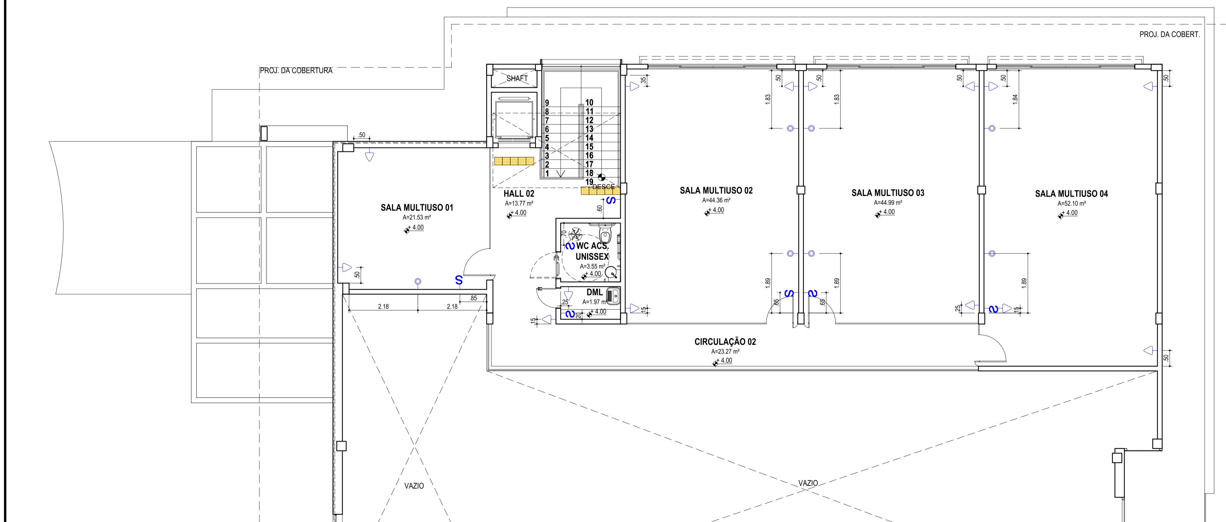
2 PLANTA 1º PAVIMENTO - PONTOS ELÉTRICOS ESCALA .....1/75
