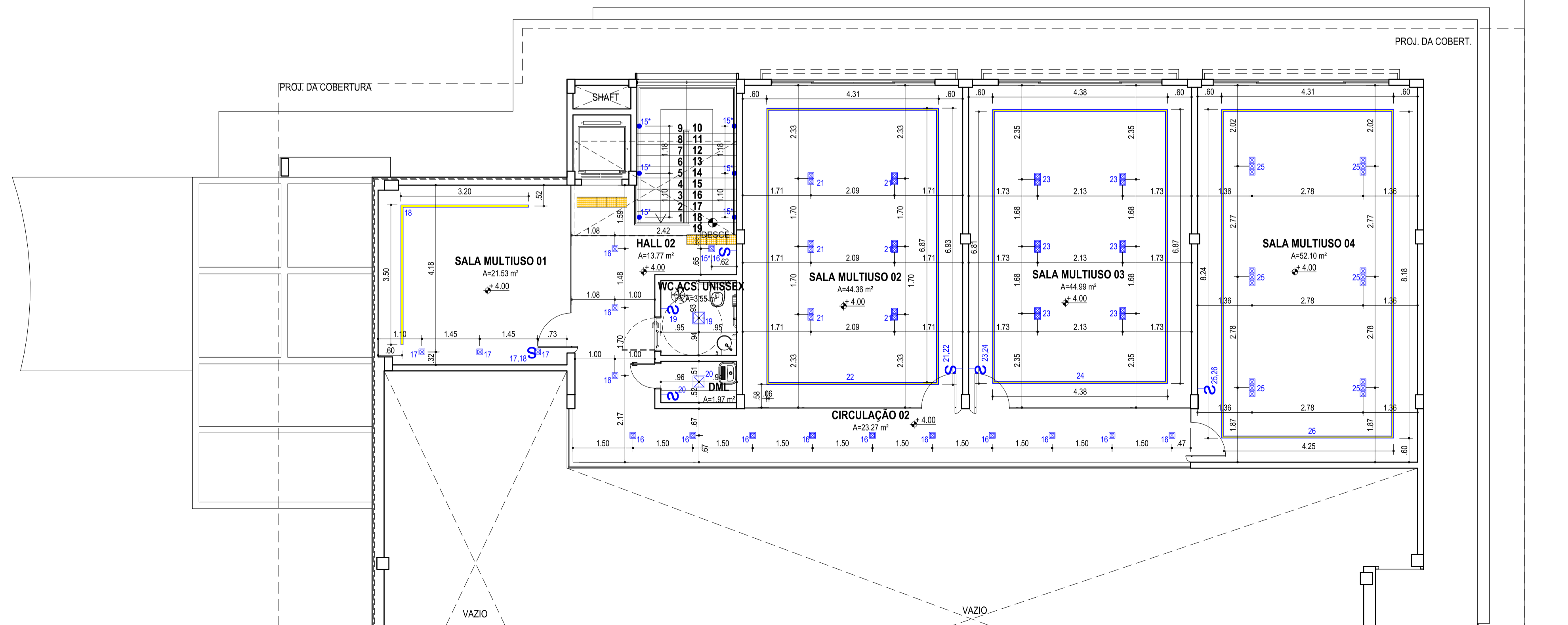
2 PLANTA 1º PAVIMENTO - PONTOS LUMINOTÉCNICOS ESCALA: 1/75
