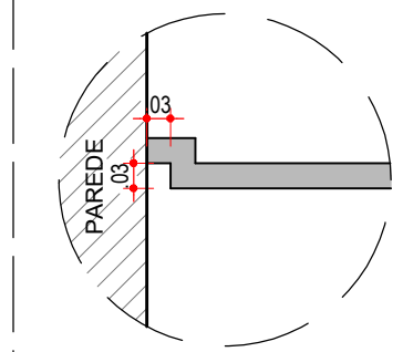
DET.01 ESCALA: 1/10
