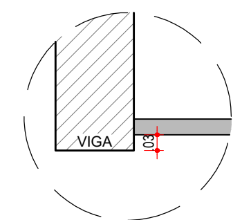
DET.02 ESCALA: 1/10
